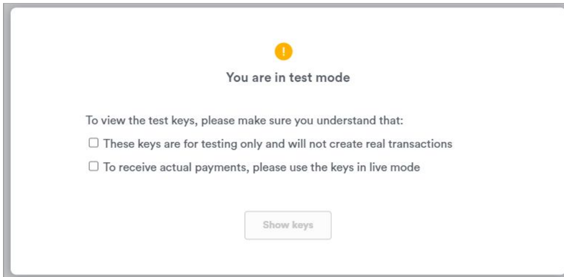
Fig. 5: Pop-up Message
